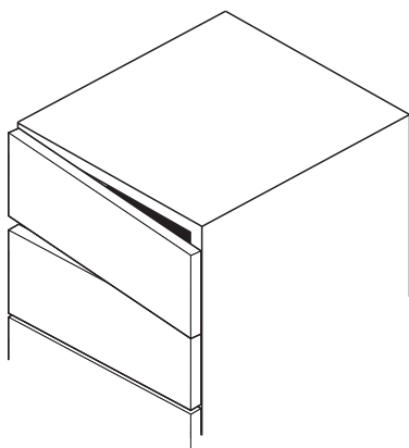
Turn the wheel to adjust the drawer height (+/-2mm). Tourner la molette pour ajuster la hauteur du tiroir (+/-2mm).
